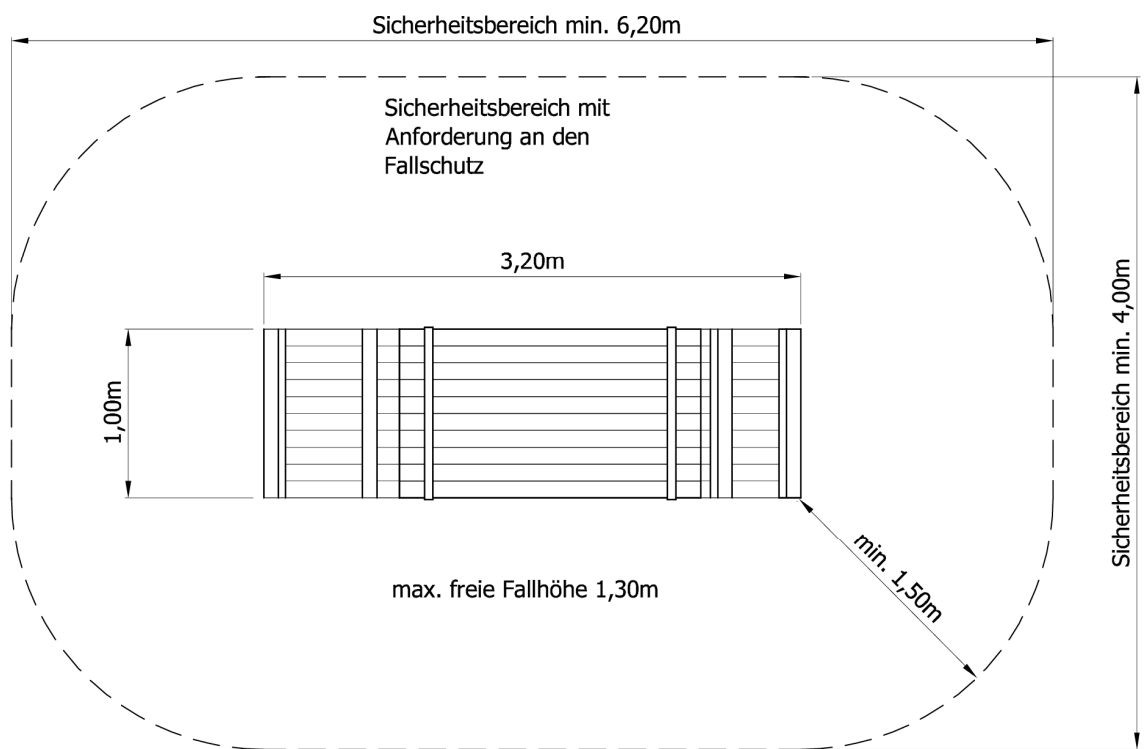
Draufsicht
