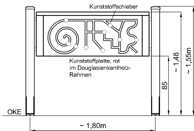
Variante mit Pfostenschuhen
