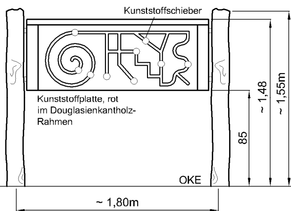
Variante mit Robinienpfosten
