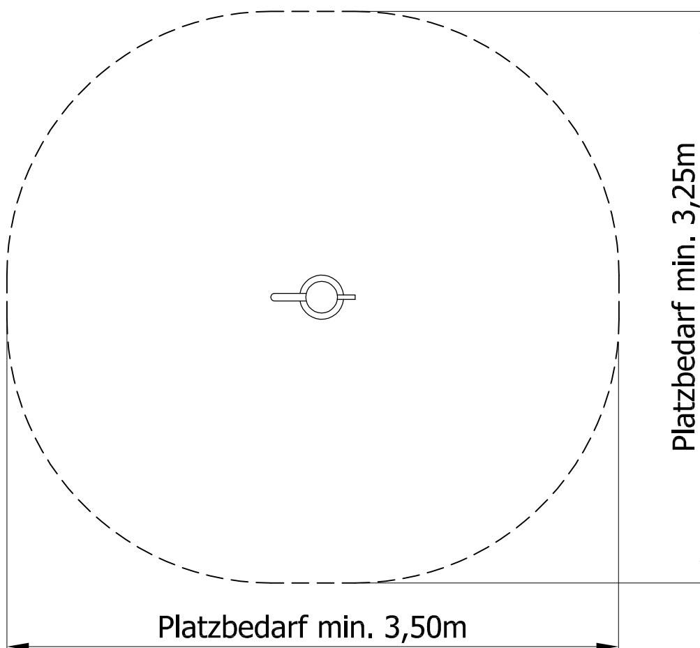
Draufsicht
