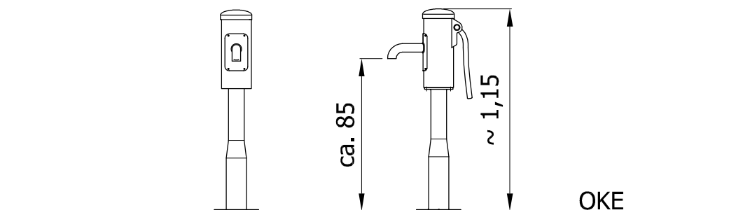
Ansicht
