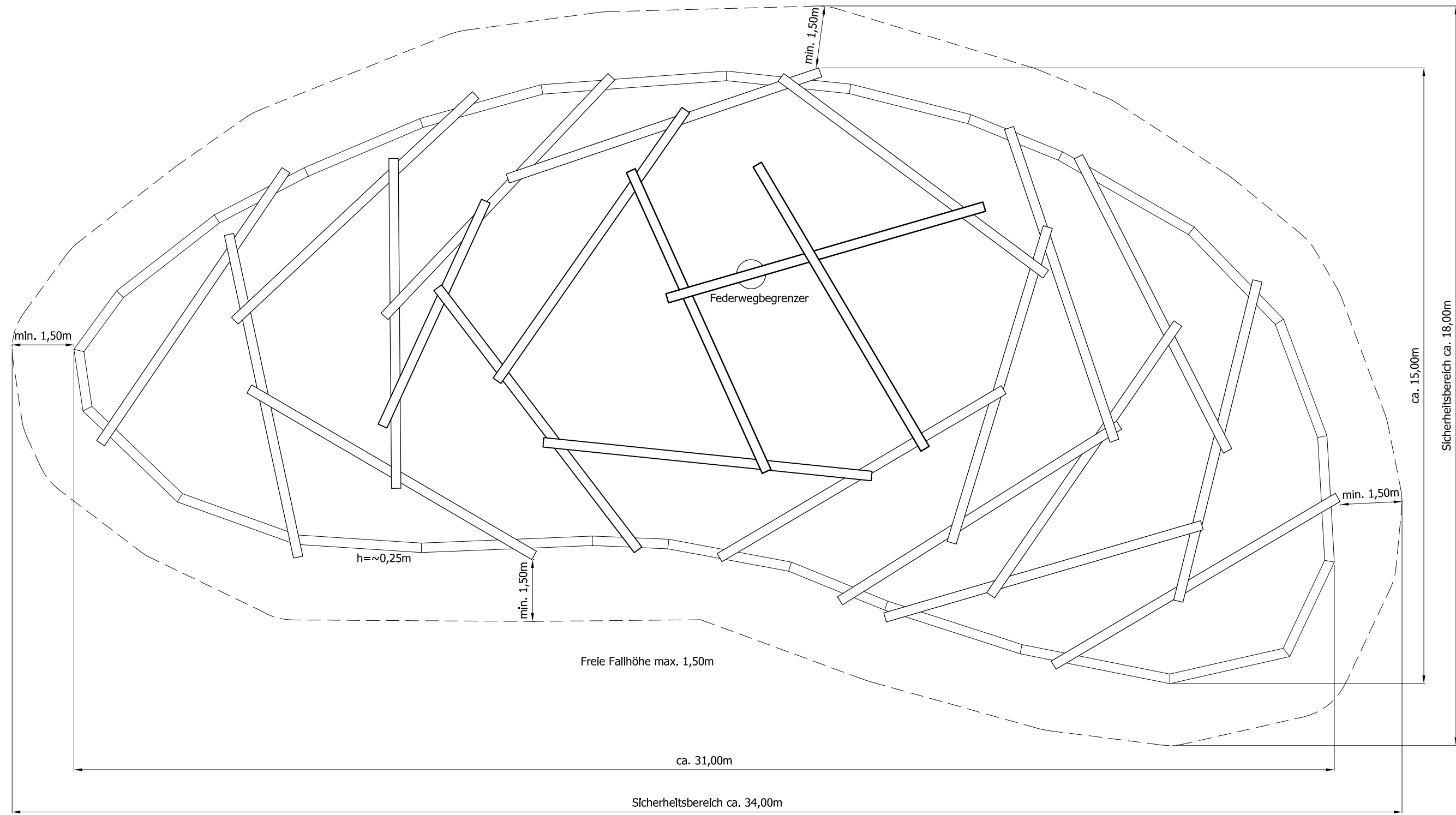
Draufsicht
