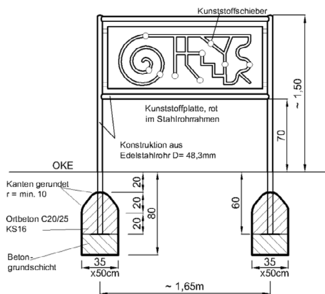
Variante in Stahlrohrrahmen
