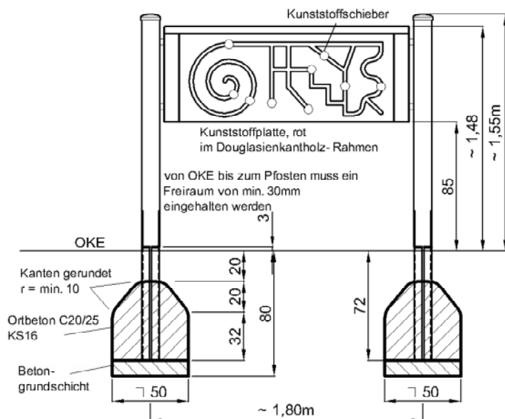
Variante mit Pfostenschuhen
