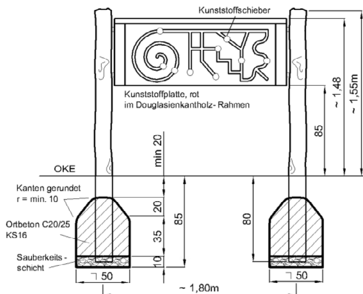
Variante mit Robinienpfosten
