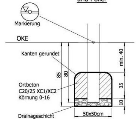
Fundamentschnitt Robiniererdeinbau Sandspieltisch und Poller
