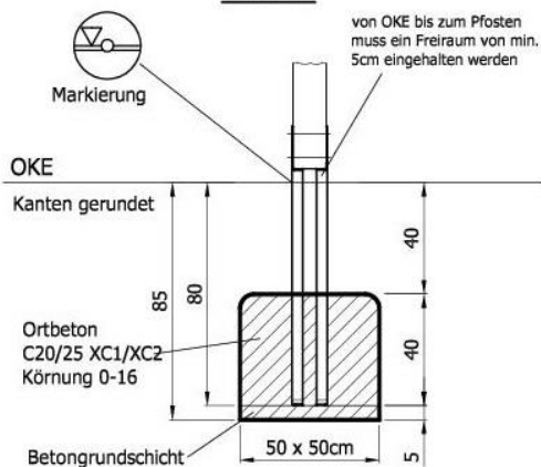
4 Stück Fundamentschnitt Pfostenschuheinbau F60x800
