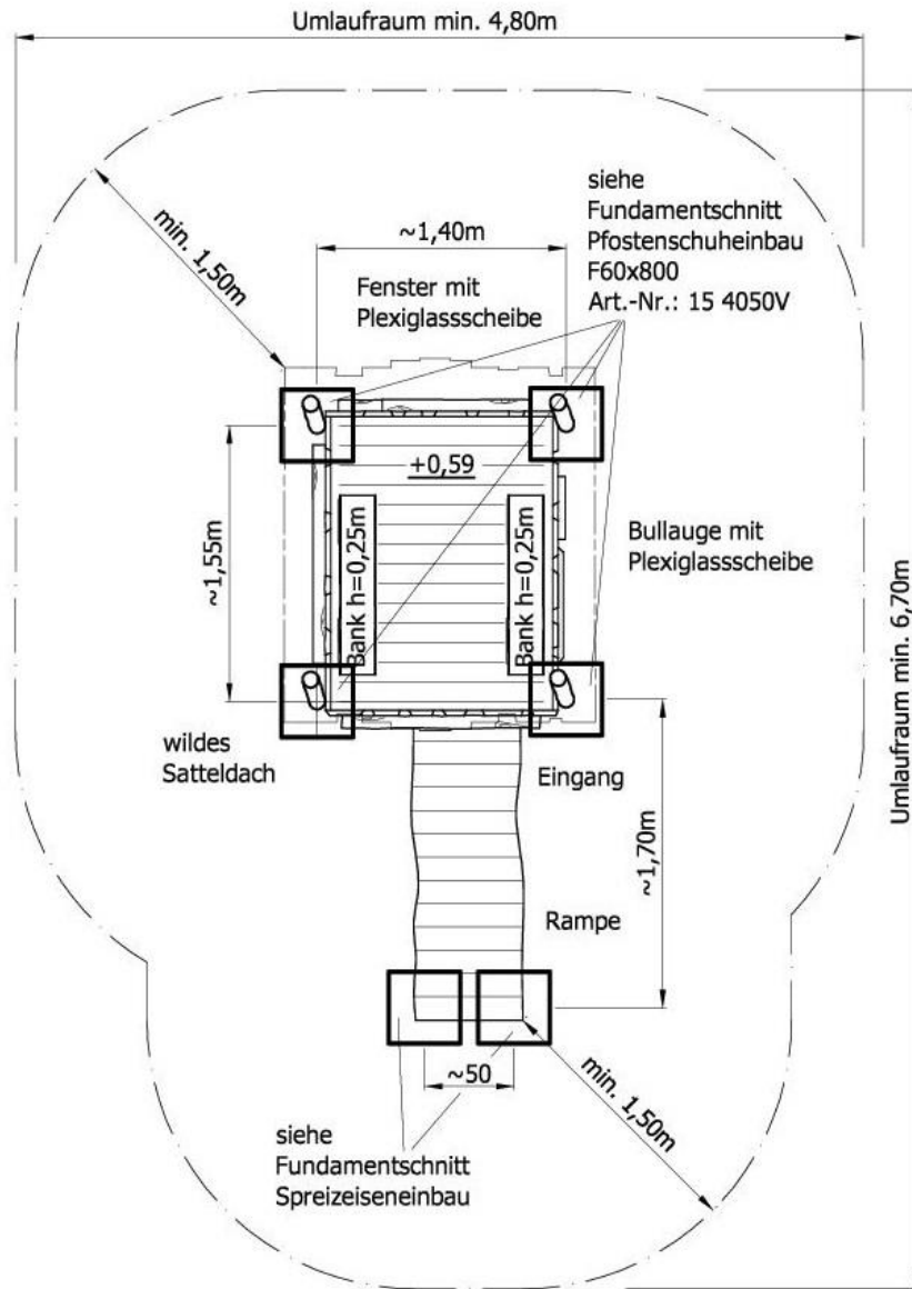
2 Stück Spreizeiseneinbau Rampe und Leiter
