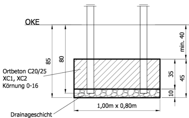
① Fundamentschnitt Fass
