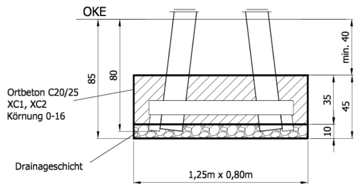
② Fundamentschnitt Wackelfass
