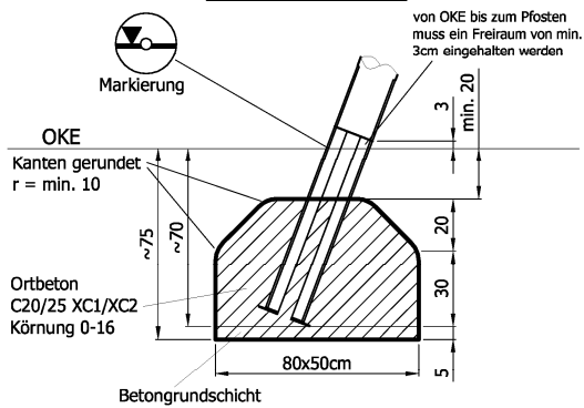
Fundamentschnitt Pfostenschuheinbau
