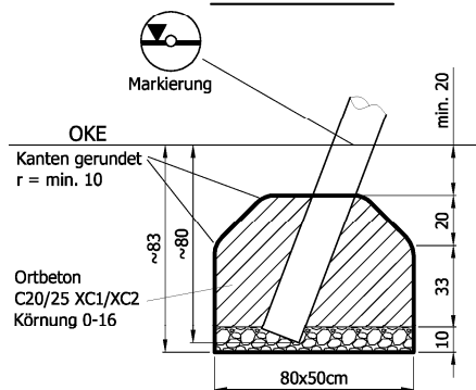
Fundamentschnitt Pfostenschuheinbau
