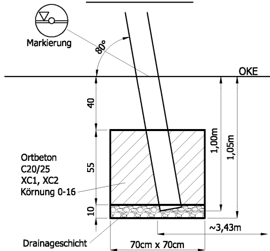
Fundamentschnitt Robinienerdeinbau
