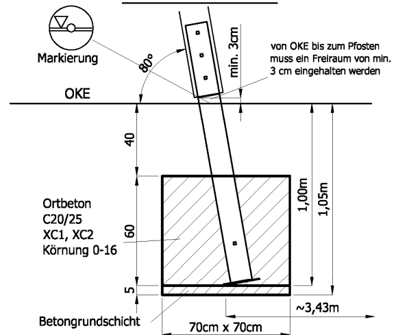
Fundamentschnitt Pfostenschuheinbau
