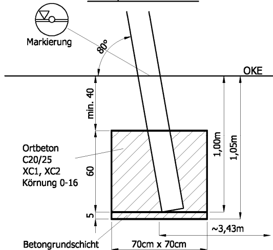
Fundamentschnitt Stahlpfosteneinbau
